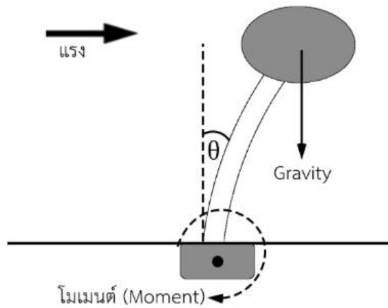
ภาพที่ 24 พฤติกรรมของต้นไม้เมื่อเกิดแรงลมกระทำจากด้านข้าง
