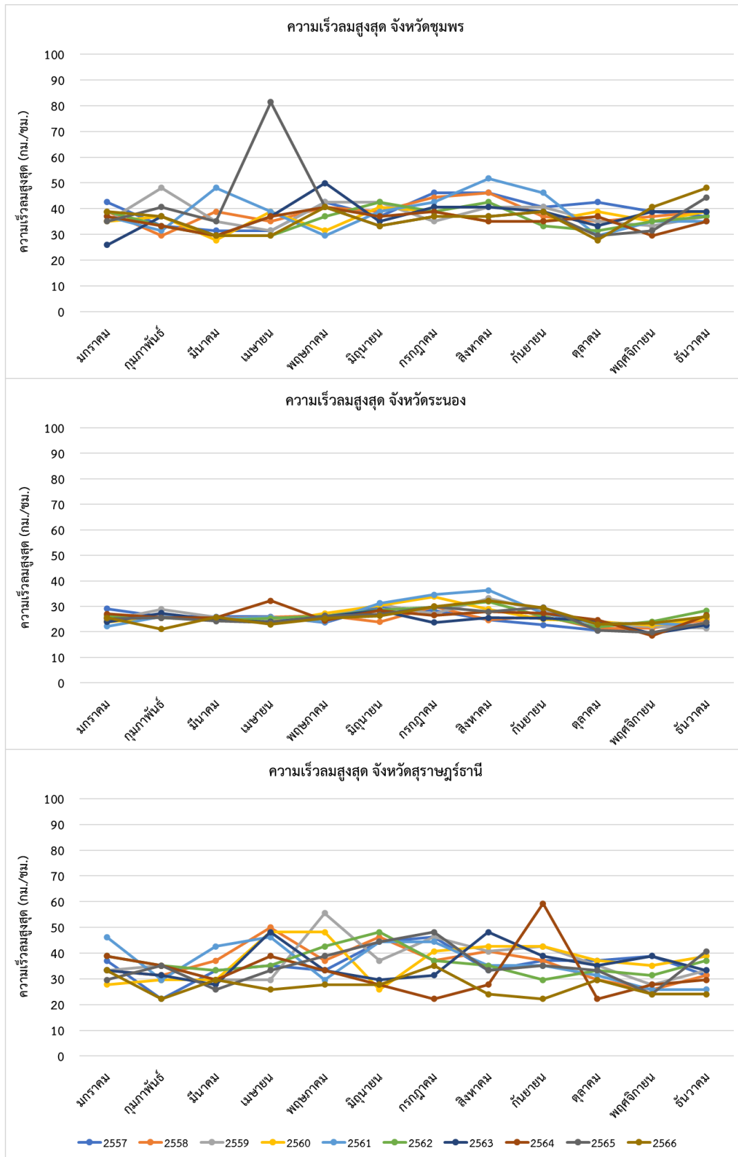
ภาพภาคผนวกที่ 27 ความเร็วลมสูงสุด (กิโลเมตร/ชั่วโมง) ระหว่างปี พ.ศ. 2557-2566 ของภาคใต้ตอนบน
