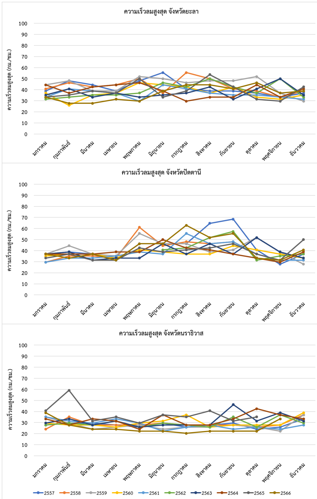
ภาพภาคผนวกที่ 29 ความเร็วลมสูงสุด (กิโลเมตร/ชั่วโมง) ระหว่างปี พ.ศ. 2557-2566 ของภาคใต้ตอนล่าง
