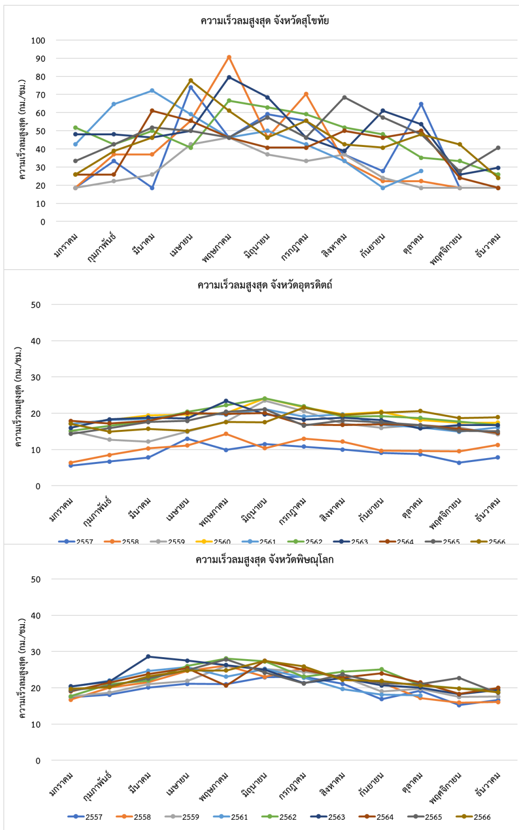
ภาพภาคผนวกที่ 25 ความเร็วลมสูงสุด (กิโลเมตร/ชั่วโมง) ระหว่างปี พ.ศ. 2557-2566 ของภาคเหนือตอนล่าง
