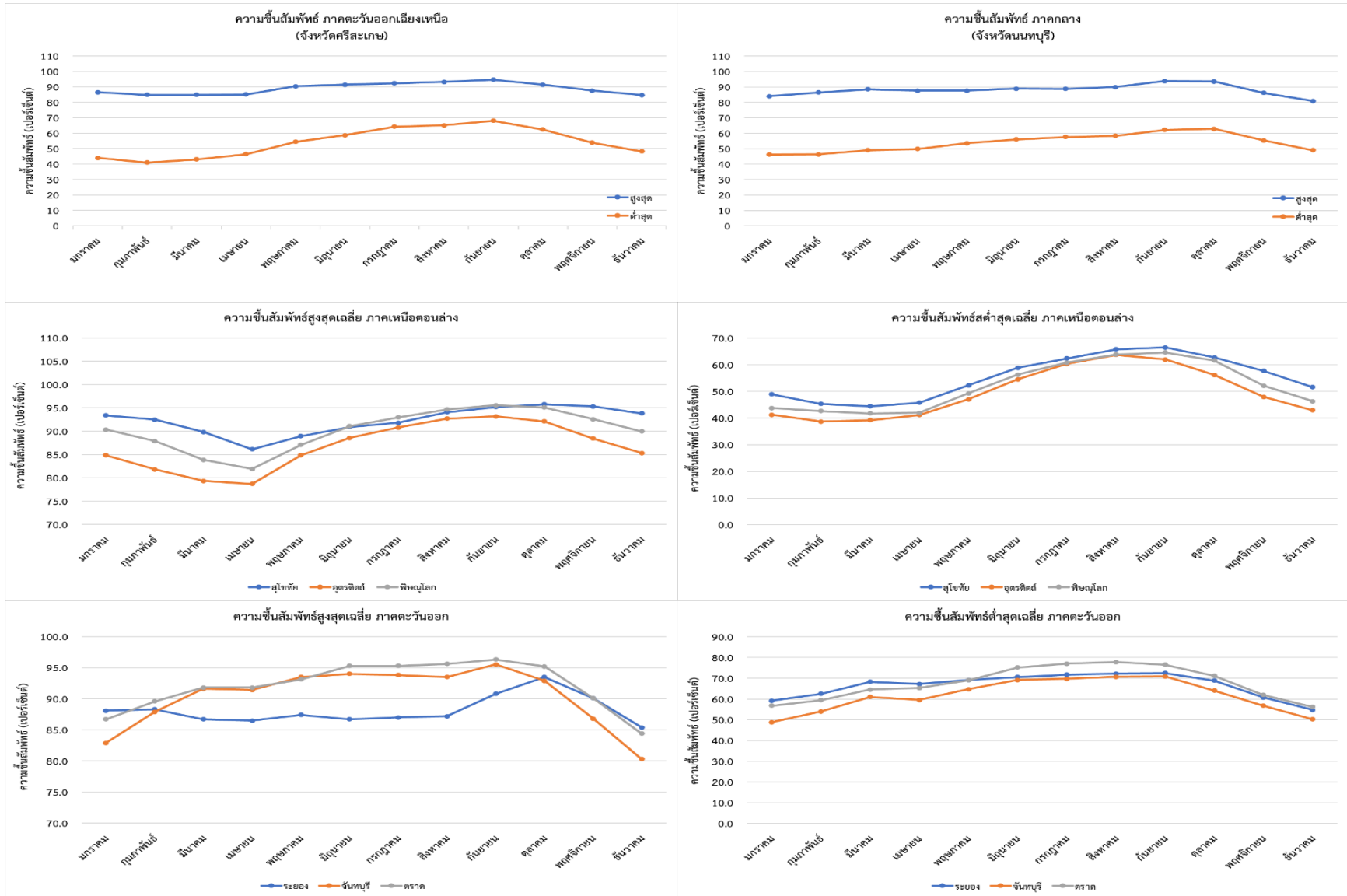
ภาพภาคผนวกที่ 22 ความชื้นสัมพัทธ์สูงสุด – ต่ำสุด (เปอร์เซ็นต์) ค่าเฉลี่ยระหว่างปี พ.ศ. 2557-2566
