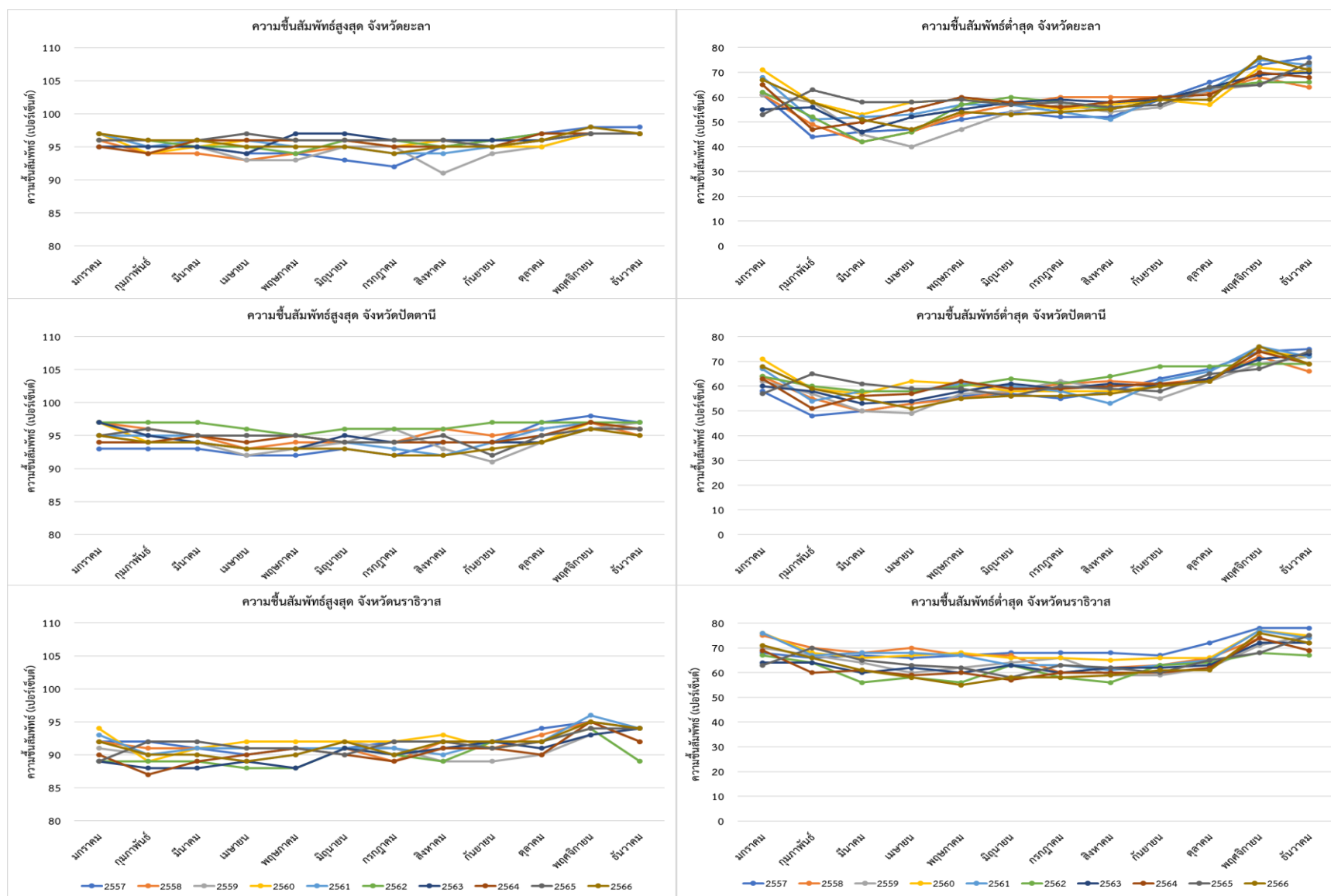
ภาพภาคผนวกที่ 21 ความชันสัมพัทธ์สูงสุด - ต่ำสุด (เปอร์เซ็นต์) ระหว่างปี พ.ศ. 2557-2566 ของภาคใต้ตอนล่าง
