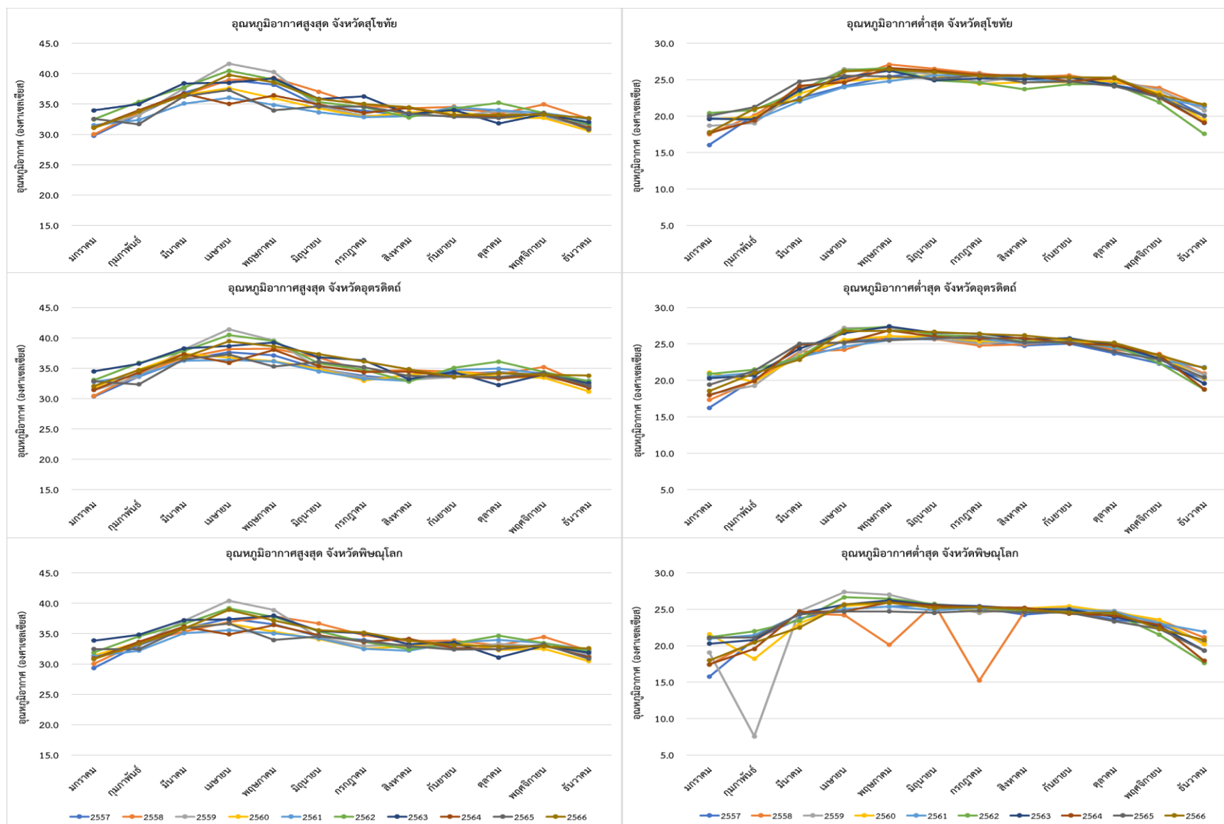
ภาพภาคผนวกที่ 9 อุณหภูมิสูงสุด – ต่ำสุด (องศาเซลเซียส) ระหว่างปี พ.ศ. 2557-2566 ของภาคเหนือตอนล่าง
