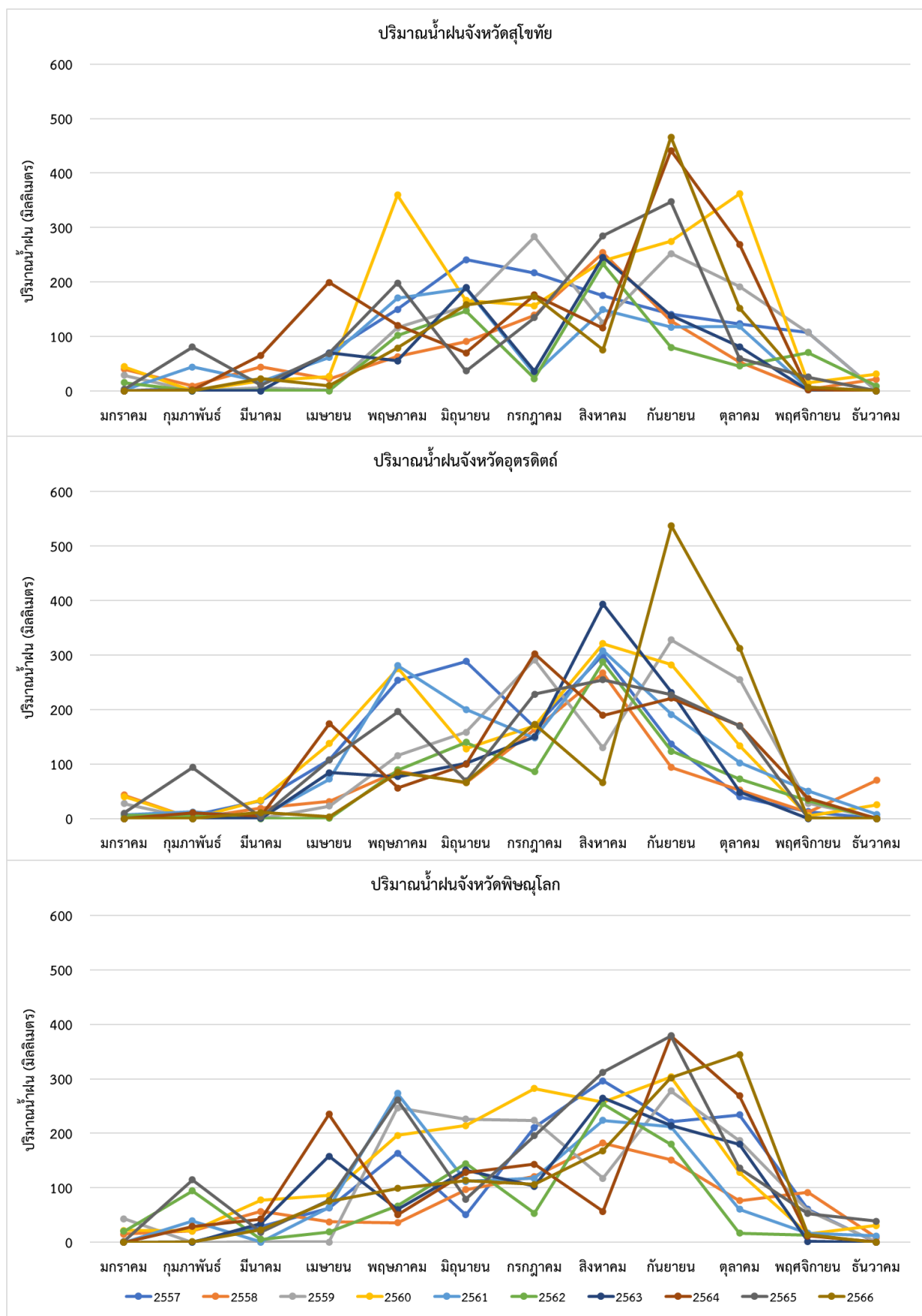
ภาพภาคผนวกที่ 2 ปริมาณน้ำฝน (มิลลิเมตร) ระหว่างปี พ.ศ. 2557-2566 ของภาคเหนือตอนล่าง
