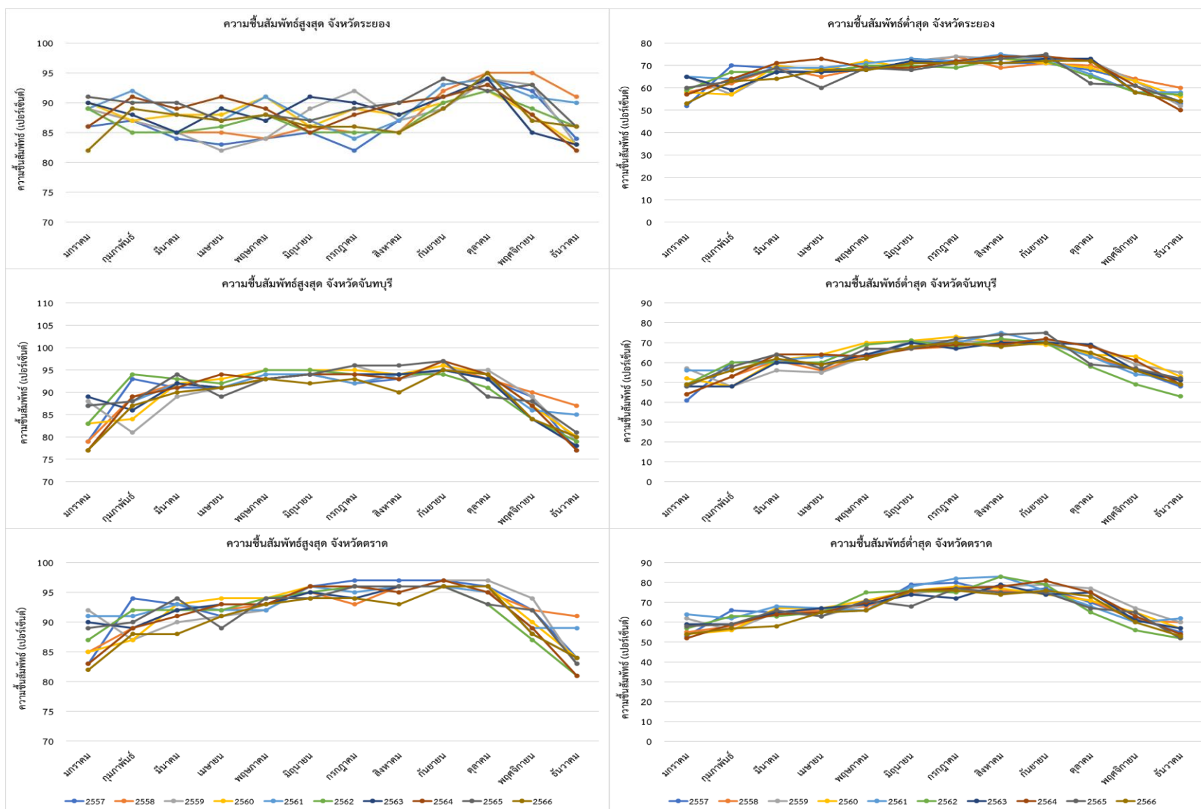
ภาพภาคผนวกที่ 18 ความชื้นสัมพัทธ์สูงสุด - ต่ำสุด (เปอร์เซ็นต์) ระหว่างปี พ.ศ. 2557-2566 ของภาคตะวันออก
