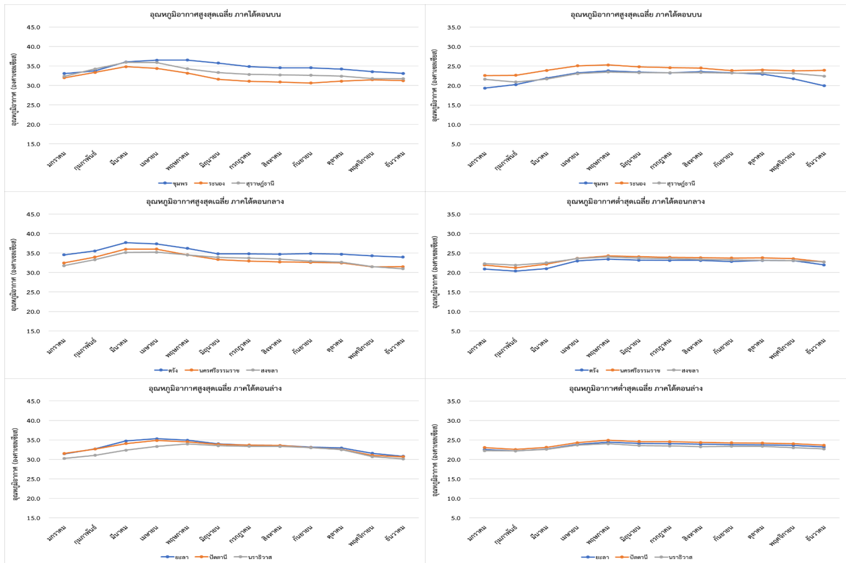
ภาพภาคผนวกที่ 15 กราฟแสดงอุณหภูมิสูงสุด – ต่ำสุด (องศาเซลเซียส) ค่าเฉลี่ยระหว่างปี พ.ศ. 2557-2566 ในพื้นที่ปลูกทุเรียน
