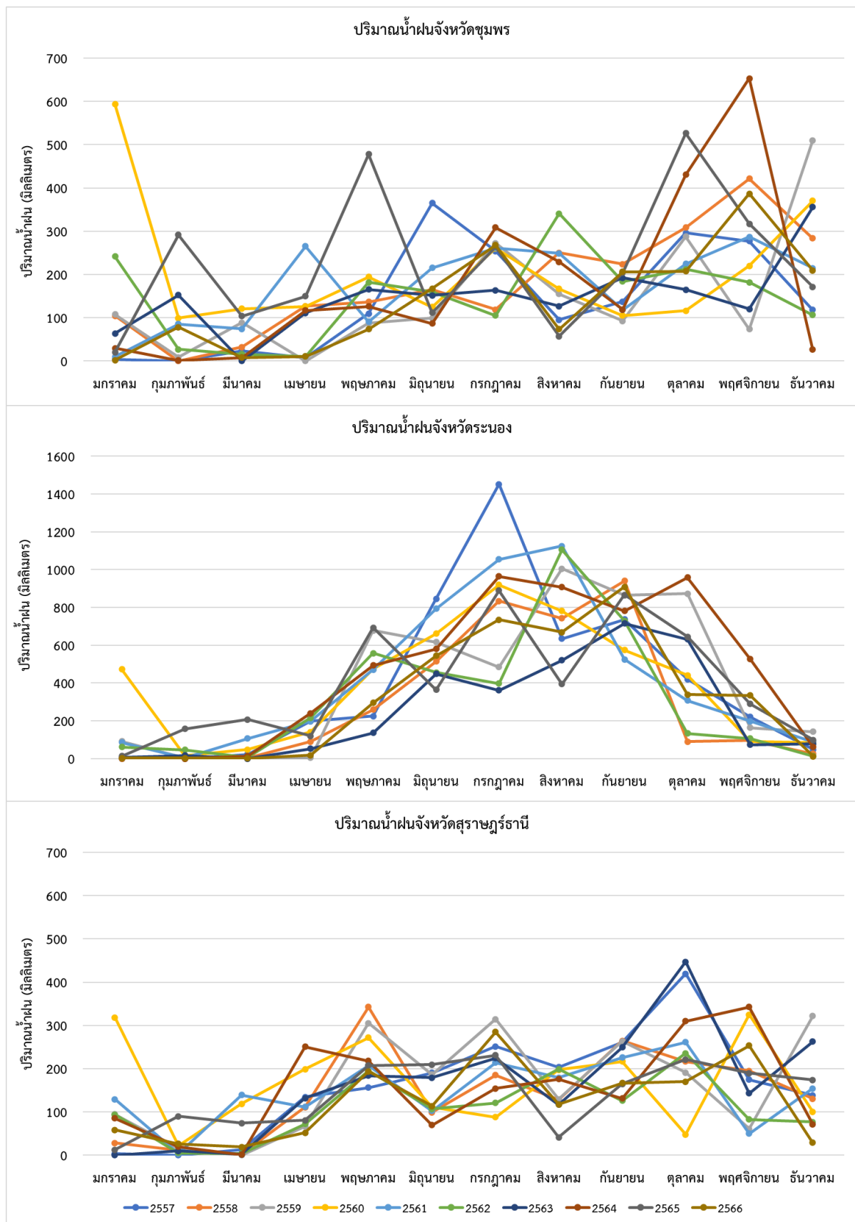
ภาพภาคผนวกที่ 4 ปริมาณน้ำฝน (มิลลิเมตร) ฝนระหว่างปี พ.ศ. 2557-2566 ของภาคใต้ตอนบน
