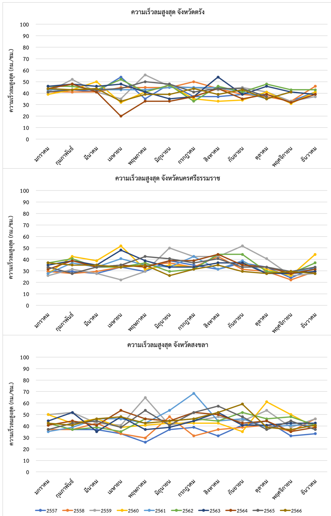
ภาพภาคผนวกที่ 28 ความเร็วลมสูงสุด (กิโลเมตร/ชั่วโมง) ระหว่างปี พ.ศ. 2557-2566 ของภาคใต้ตอนกลาง
