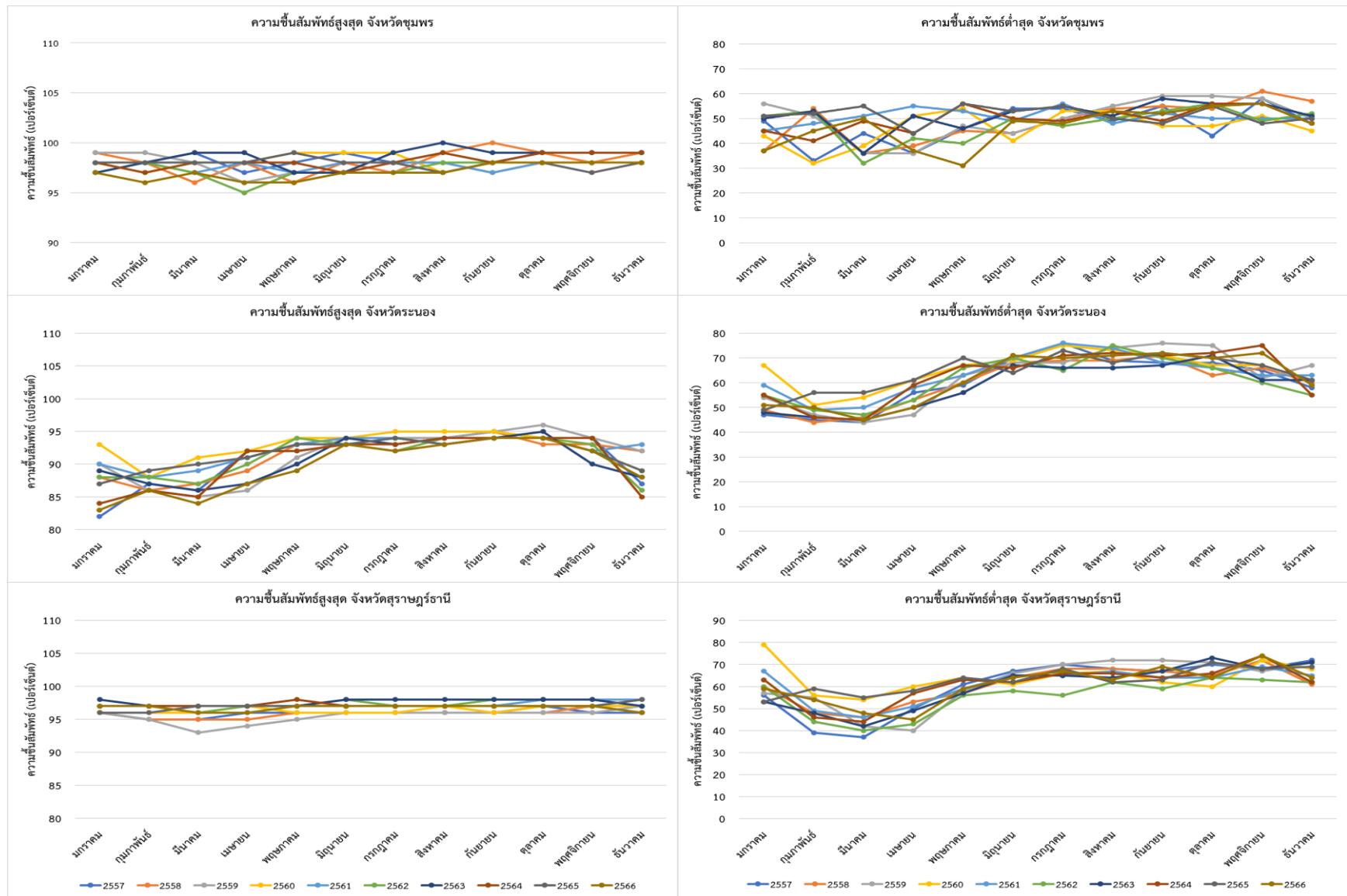
ภาพภาคผนวกที่ 19 ความชื้นสัมพัทธ์สูงสุด - ต่ำสุด (เปอร์เซ็นต์) ระหว่างปี พ.ศ. 2557-2566 ของภาคใต้ตอนบน
