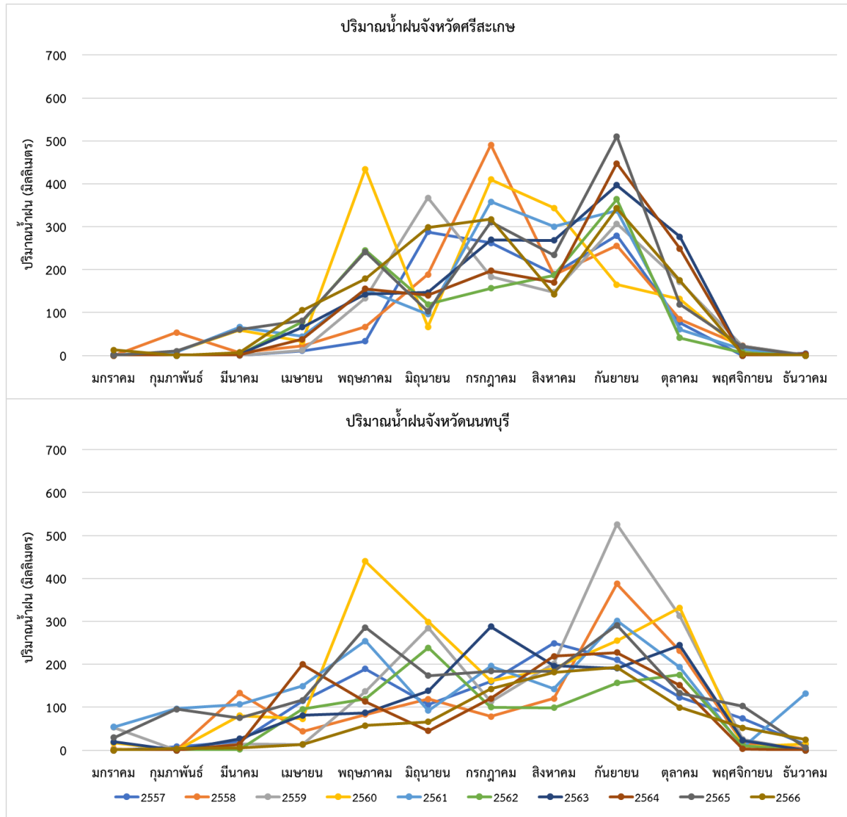
ภาพภาคผนวกที่ 1 ปริมาณน้ำฝน (มิลลิเมตร) ระหว่างปี พ.ศ. 2557-2566 ของจังหวัดศรีสะเกษและนนทบุรี
