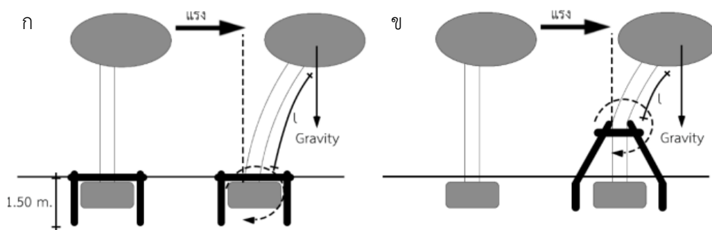
ภาพที่ 25 พฤติกรรมของไม้ค้ำระบบรากเทียม และไม้ค้ำแบบกระโจม
