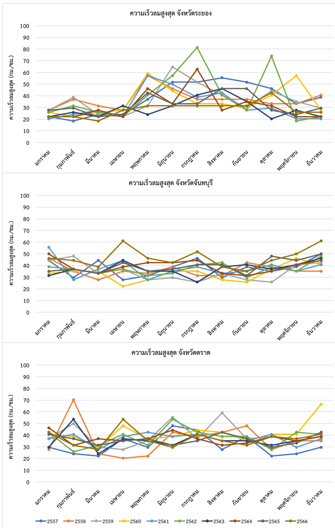
ภาพภาคผนวกที่ 26 ความเร็วลมสูงสุด (กิโลเมตร/ชั่วโมง) ระหว่างปี พ.ศ. 2557-2566 ของภาคตะวันออก
