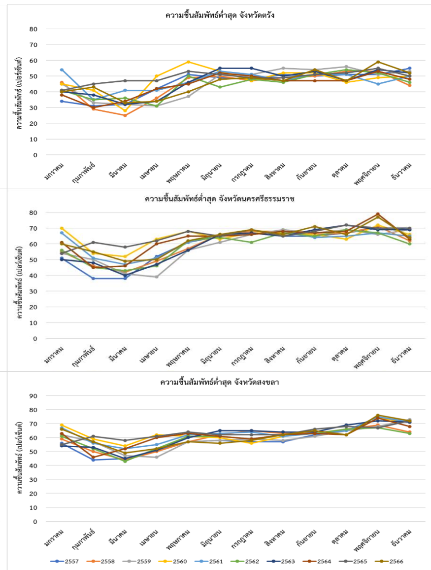
ภาพภาคผนวกที่ 20 ความชันสัมพัทธ์สูงสุด - ต่ำสุด (เปอร์เซ็นต์) ระหว่างปี พ.ศ. 2557-2566 ของภาคใต้ตอนกลาง
