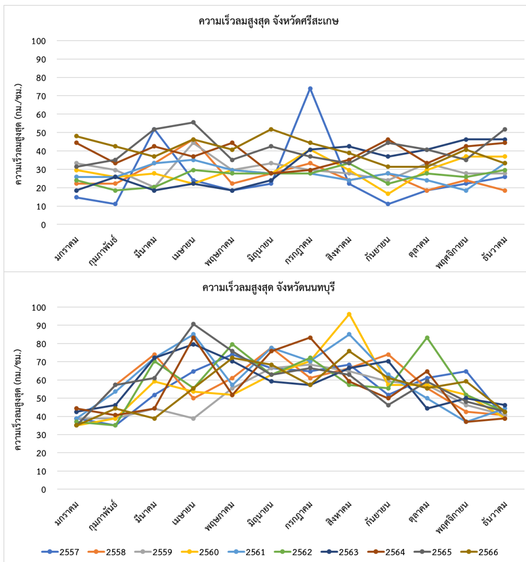
ภาพภาคผนวกที่ 24 ความเร็วสูงสุด (กิโลเมตร/ชั่วโมง) ระหว่างปี พ.ศ. 2557-2566 ของจังหวัดศรีสะเกษ และ นนทบุรี
