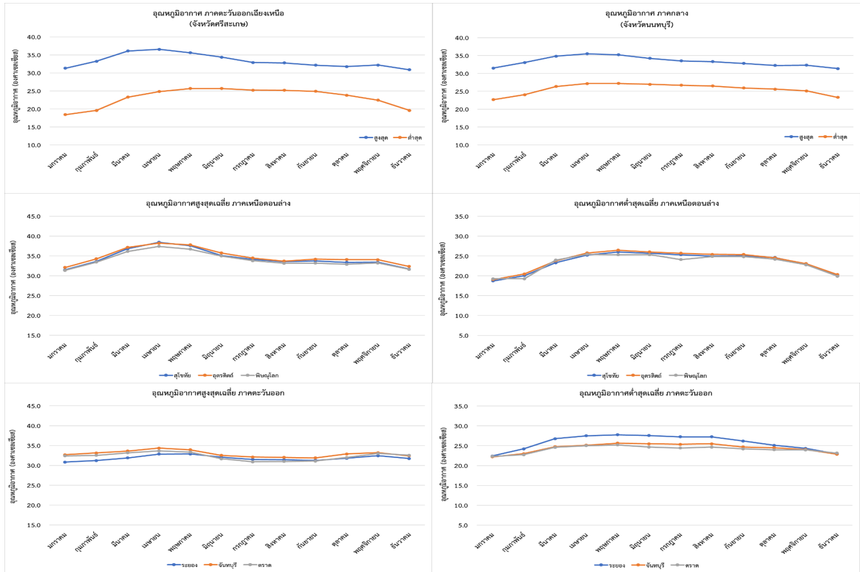
ภาพภาคผนวกที่ 14 กราฟแสดงอุณหภูมิสูงสุด – ต่ำสุด (องศาเซลเซียส) ค่าเฉลี่ยระหว่างปี พ.ศ. 2557-2566 ในพื้นที่ปลูกทุเรียน
