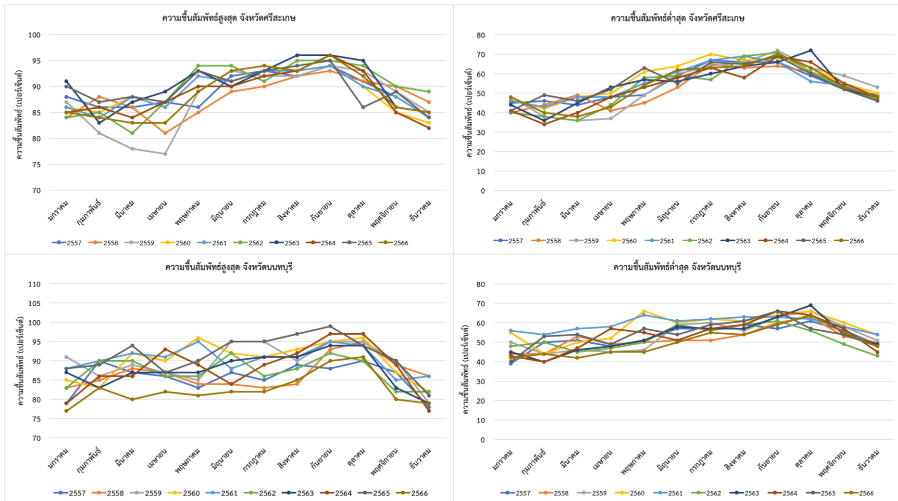
ภาพภาคผนวกที่ 16 ความชื้นสัมพัทธ์สูงสุด - ต่ำสุด (เปอร์เซ็นต์) ระหว่างปี พ.ศ. 2557-2566 ของจังหวัดศรีสะเกษและนนทบุรี
