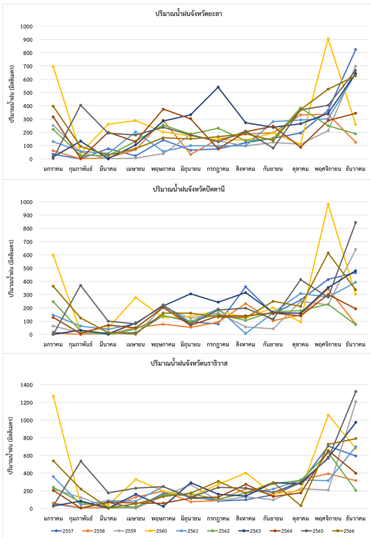
ภาพภาคผนวกที่ 6 ปริมาณน้ำฝน (มิลลิเมตร) ฝนระหว่างปี พ.ศ. 2557-2566 ของภาคใต้ตอนล่าง
