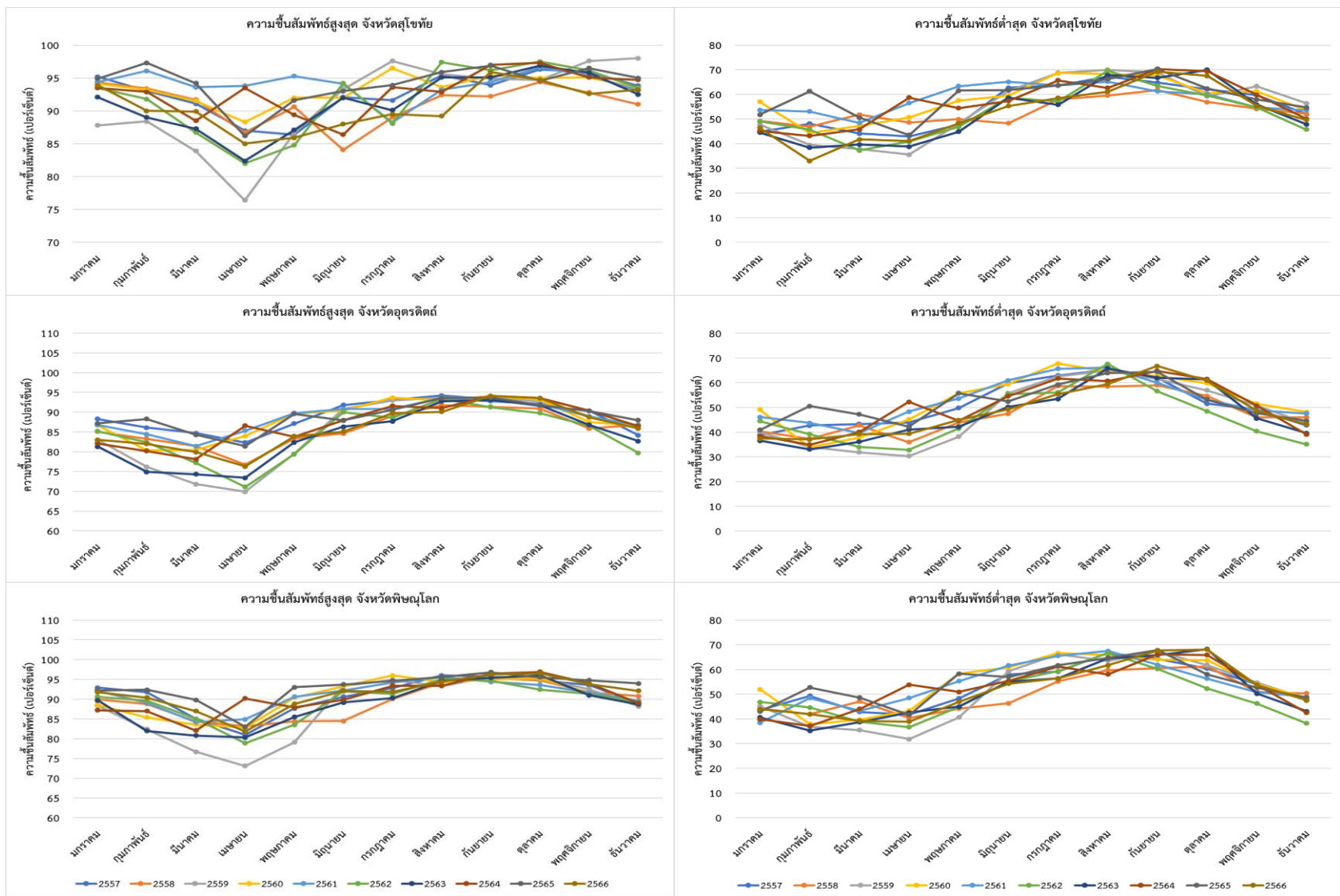
ภาพภาคผนวกที่ 17 ความชื้นสัมพัทธ์สูงสุด - ต่ำสุด (เปอร์เซ็นต์) ระหว่างปี พ.ศ. 2557-2566 ของภาคเหนือตอนล่าง
