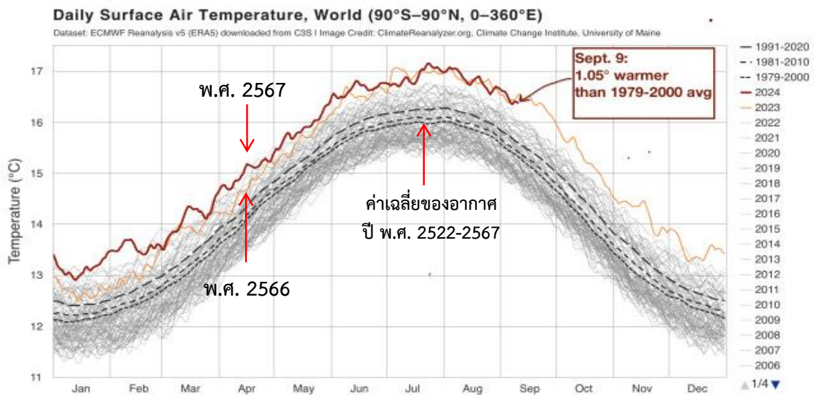
ภาพที่ 1 กราฟอุณหภูมิเฉลี่ยของอากาศรายวันที่ระดับมาตรฐาน 2 เมตรจากผิวโลก (องศาเซลเซียส) ระหว่างปี พ.ศ. 2522-2567 ที่มา: Daily Surface Air Temperature, 2024
