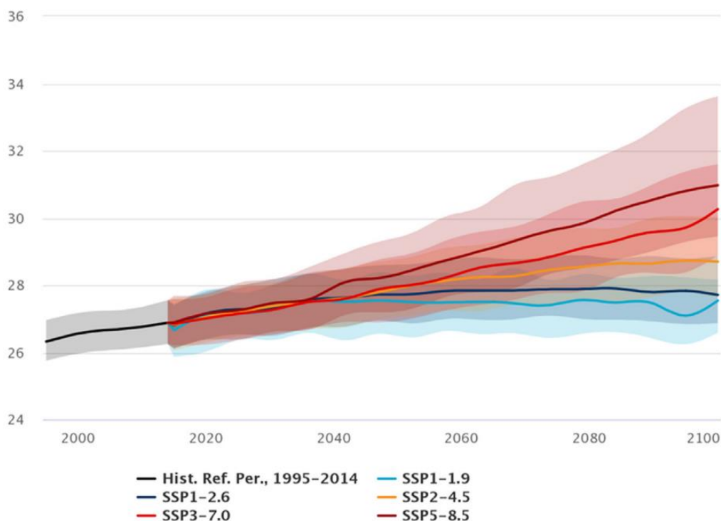
ภาพที่ 2 อุณหภูมิรายปีเฉลี่ยในอนาคตจำแนกตามภาพฉายการเปลี่ยนแปลงสภาพภูมิอากาศ ที่มา: The World Bank, 2022
