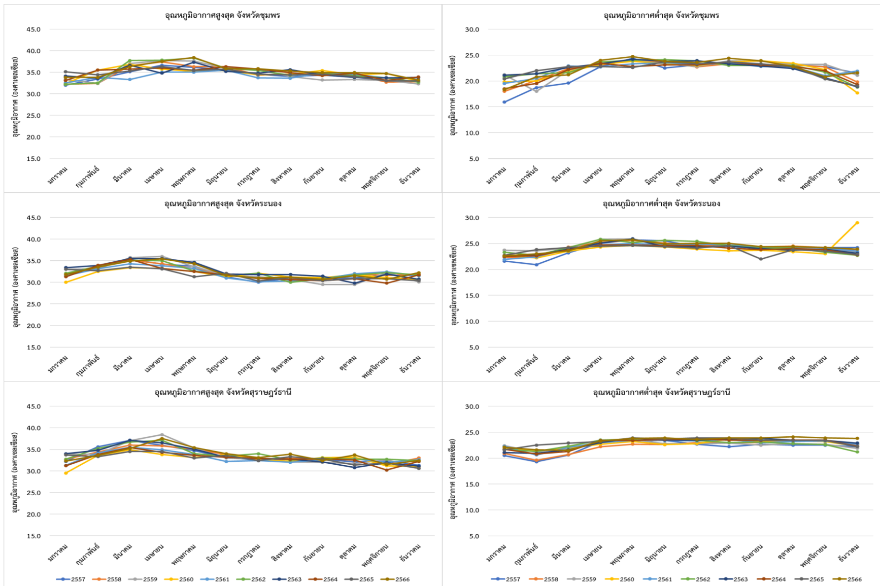
ภาพภาคผนวกที่ 11 อุณหภูมิสูงสุด – ต่ำสุด (องศาเซลเซียส) ระหว่างปี พ.ศ. 2557-2566 ของภาคใต้ตอนบน
