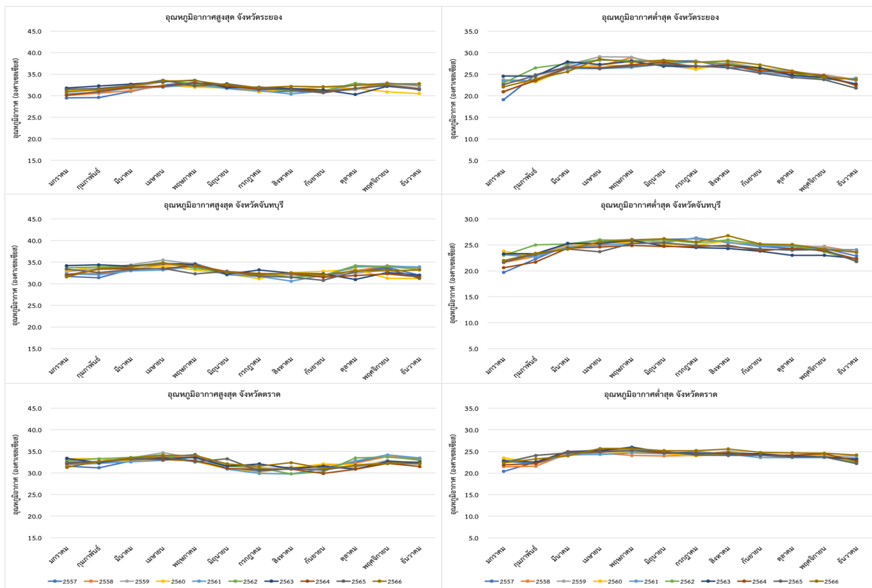
ภาพภาคผนวกที่ 10 อุณหภูมิสูงสุด – ต่ำสุด (องศาเซลเซียส) ระหว่างปี พ.ศ. 2557-2566 ของภาคตะวันออก
