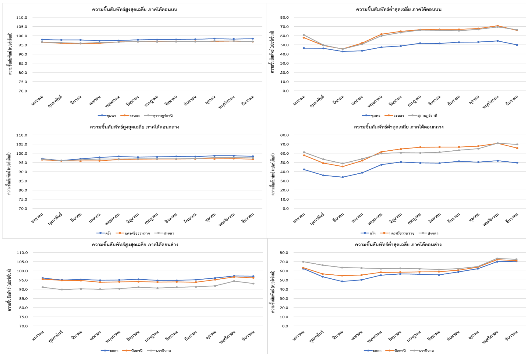
ภาพภาคผนวกที่ 23 ความเข้มข้นสัมพัทธ์สูงสุด – ต่ำสุด (เปอร์เซ็นต์) ค่าเฉลี่ยระหว่างปี พ.ศ. 2557-2566
