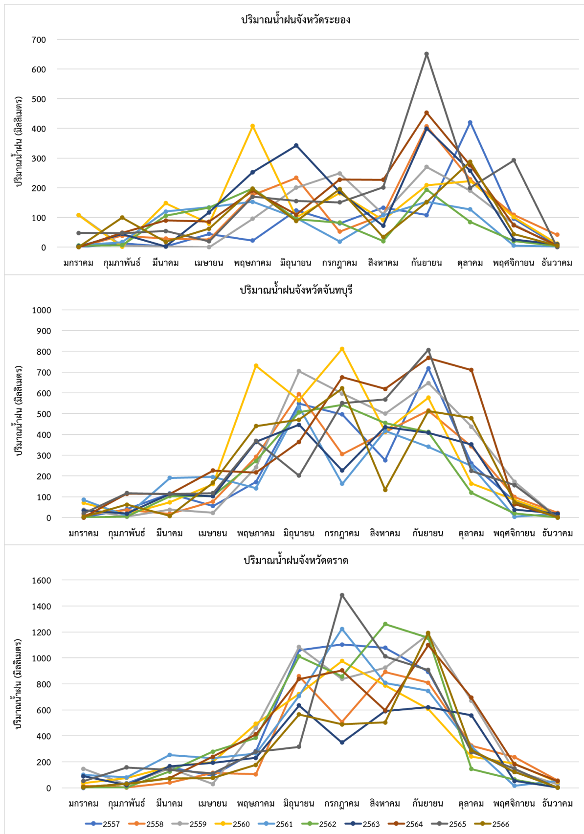
ภาพภาคผนวกที่ 3 ปริมาณน้ำฝน (มิลลิเมตร) ระหว่างปี พ.ศ. 2557-2566 ของภาคตะวันออก
