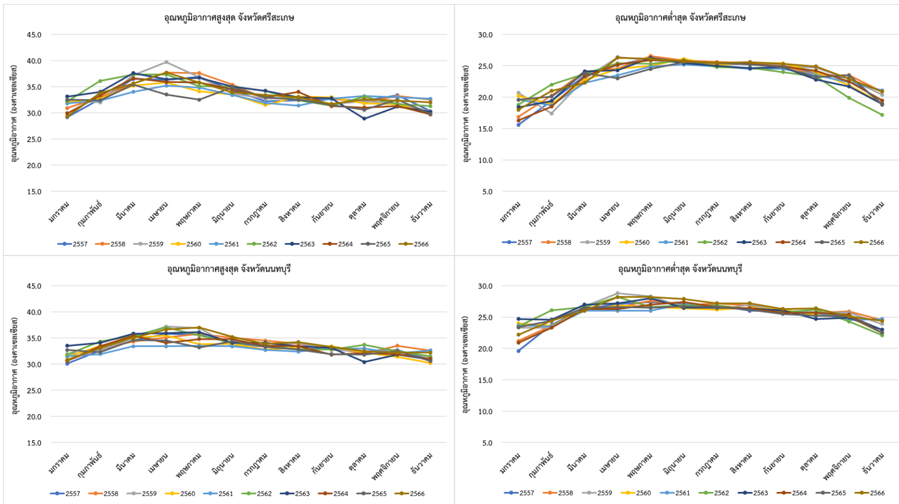
ภาพภาคผนวกที่ 8 อุณหภูมิสูงสุด – ต่ำสุด (องศาเซลเซียส) ระหว่างปี พ.ศ. 2557-2566 ของจังหวัดศรีสะเกษและนนทบุรี
