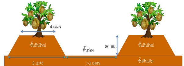
ภาพที่ 1 รูปตามขวางการปลูกทุเรียนแบบยกโคก
