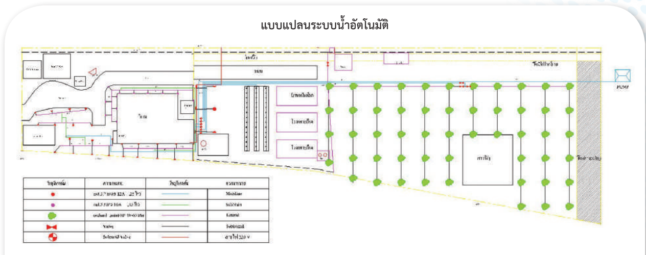
ภาพที่ 8 ตัวอย่างแผนผังที่วัดระยะโดยใช้เทปวัดระยะ
