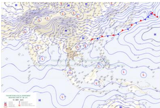
แผนที่อากาศผิวพื้น วันที่ 19 พฤษภาคม 2568 เวลา 07:00 น.
