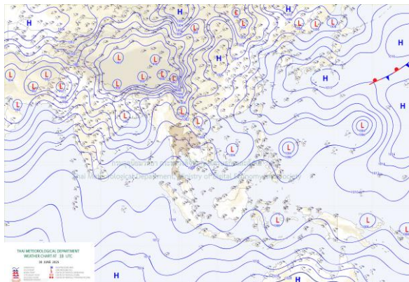
แผนที่อากาศผิวพื้นวันที่ 1 กรกฎาคม 2568 เวลา 07:00 น.
