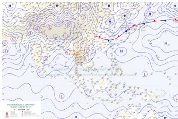
แผนที่อากาศผิวพื้นวันที่ 10 กันยายน 2568 เวลา 07:00 น.
