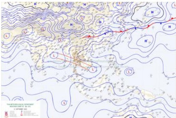
แผนที่อากาศผิวพื้นวันที่ 12 กันยายน 2568 เวลา 07:00 น.
