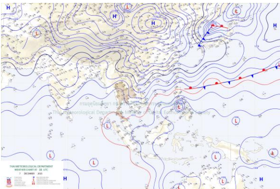
แผนที่อากาศผิวพื้นวันที่ 8 ธันวาคม 2568 เวลา 07:00 น.
