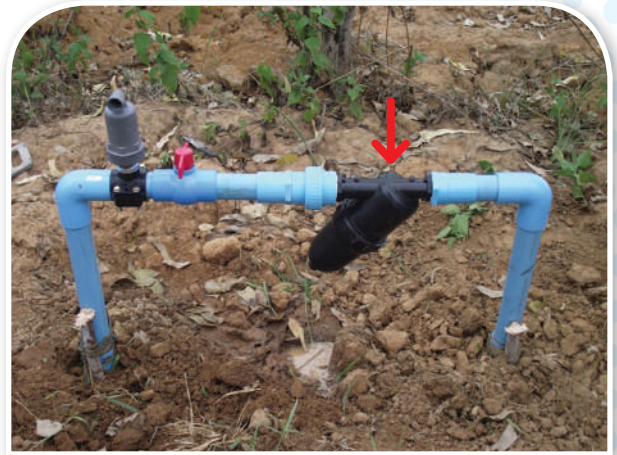
ภาพที่ 45 การติดตั้งกรองเกษตรแบบต่างๆ
