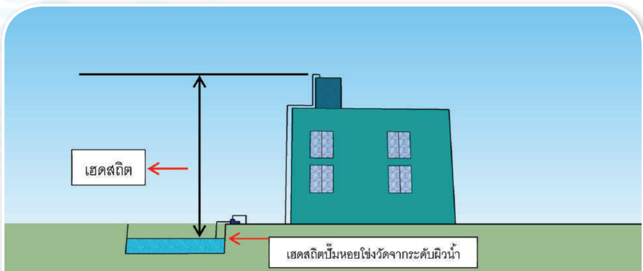
ภาพที่ 70 ตัวอย่างระดับเฮดสถิตของปั๊มหอยโข่งกรณีสูบน้ำขึ้นถังเก็บน้ำบนตึก
