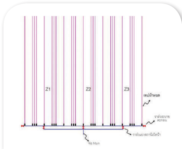
ภาพที่ 63 ตัวอย่างการแบ่งสถานีจ่ายน้ำแบบ 1 สถานีและ 3 สถานี (Z1-Z3 คือ โซนที่ 1-3)
