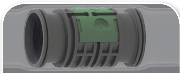
ภาพที่ 37 ภาพแสดงให้เห็นชุดปล่อยน้ำภายในท่อน้ำหยด ที่มาภาพ http://riivulix.com/products/driplines/hydropcl?change-modal=
