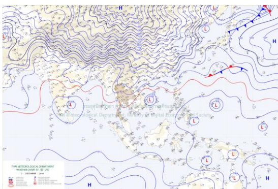
แผนที่อากาศผิวพื้นวันที่ 2 พฤศจิกายน 2568 เวลา 07:00 น.
