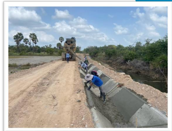
๕.๘ งานคูส่งน้ำตาดคอนกรีตแล้วเสร็จ
