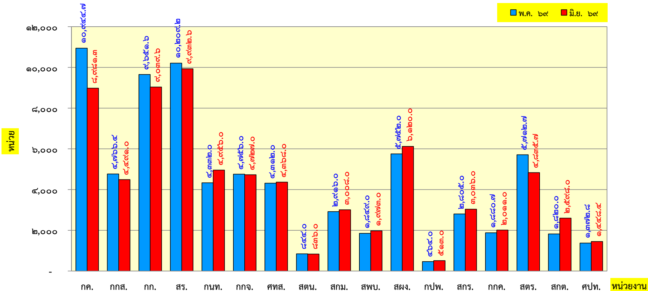
กราฟแสดงปริมาณการใช้พลังงานไฟฟ้าของหน่วยงานภายในสำนักงานปลัดกระทรวงเกษตรและสหกรณ์ เปรียบเทียบระหว่างเดือนพฤษภาคม ๒๕๖๙ กับเดือนมิถุนายน ๒๕๖๙
