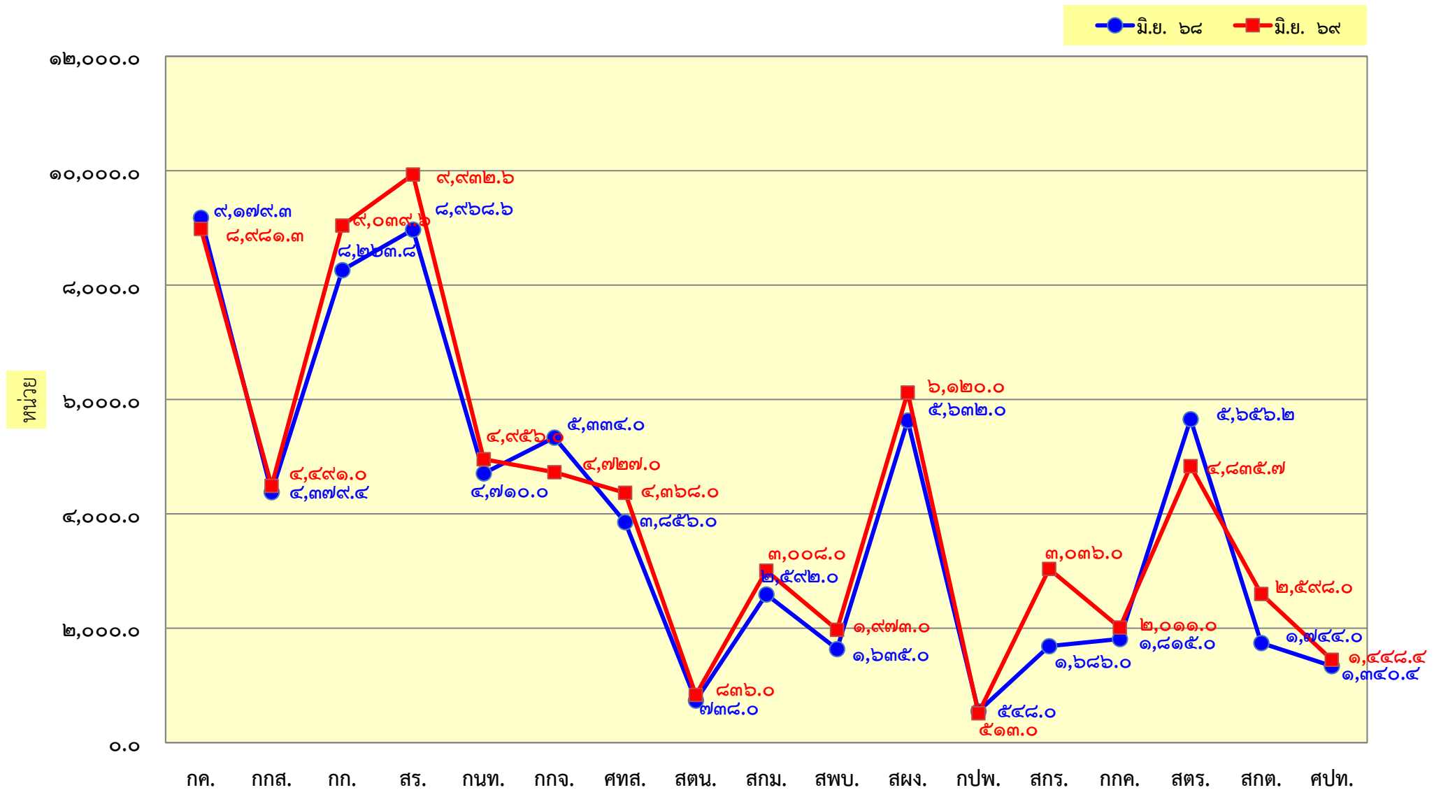
กราฟแสดงปริมาณการใช้ไฟฟ้าของหน่วยงานภายในสำนักงานปลัดกระทรวงเกษตรและสหกรณ์ เปรียบเทียบระหว่างปี พ.ศ. ๒๕๖๘ กับปี พ.ศ. ๒๕๖๙ ประจำเดือนมิถุนายน
