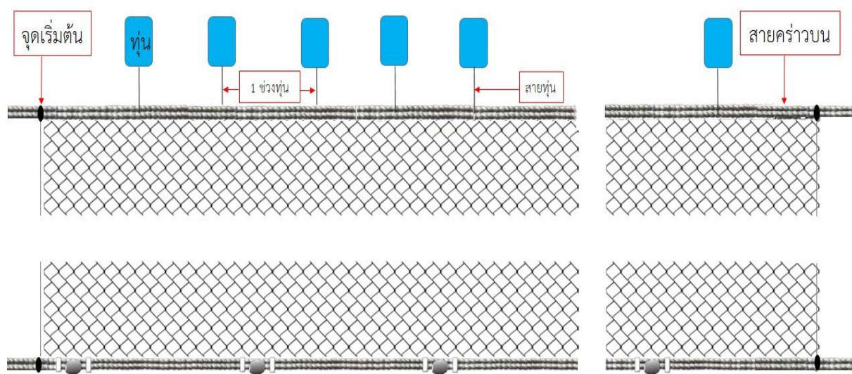
ภาพที่ ๒๔ การวัดความยาวช่วงท่อน
