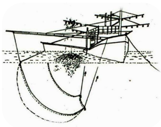
ภาพที่ ๔๕ ลักษณะของเครื่องมืออวนช้อน/ยกปลาเกะตักขณะทำการประมง (กรมประมง, ๒๕๕๙)
