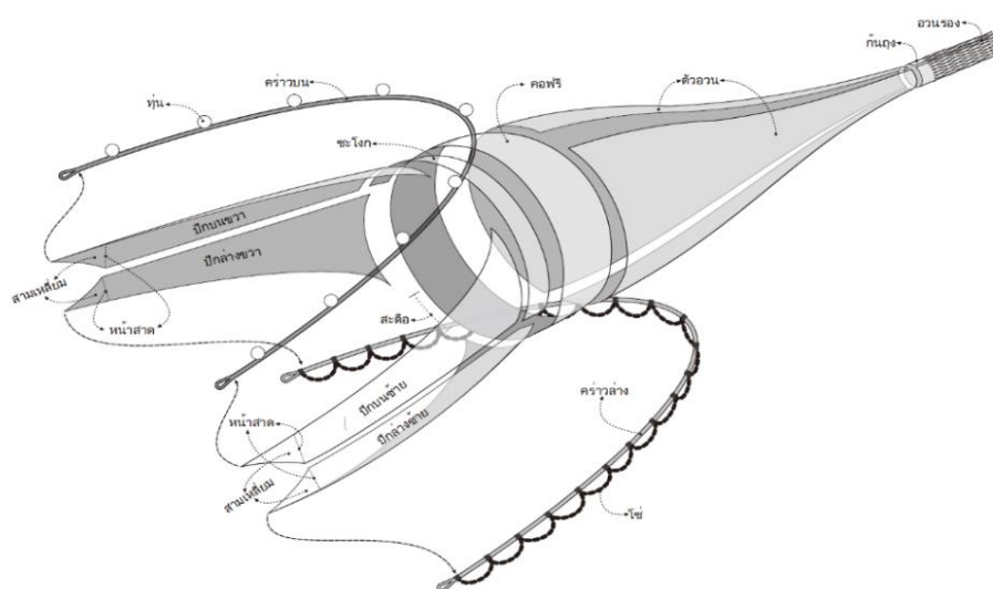
ภาพที่ ๘ ลักษณะโครงสร้างของเครื่องมืออวนลาก
