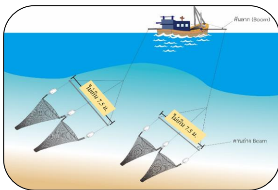
ภาพที่ ๒๒ วิธีการวัดความยาวของคันถ่าง
