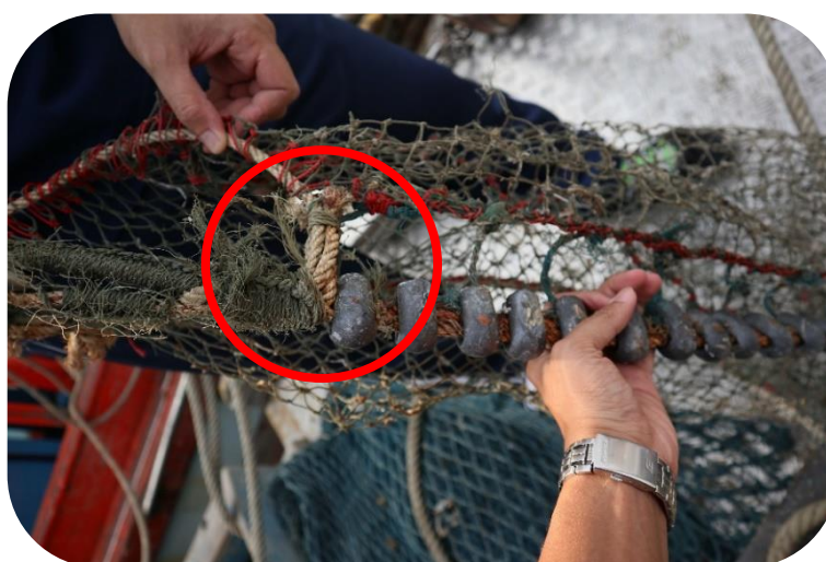
ภาพที่ ๒๓ จุดที่มีการเย็บเนื้อวนให้ติดกับเชือกคร่าวล่าง
