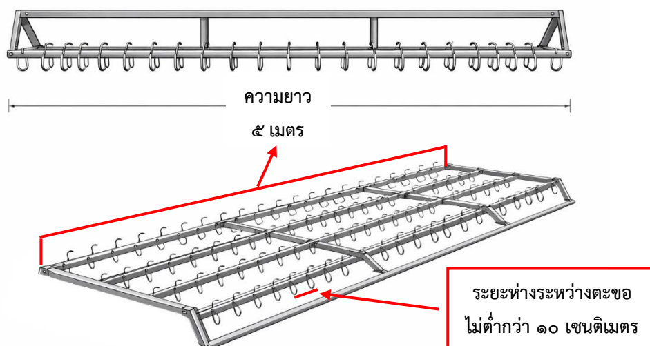
ภาพที่ ๔๑ วิธีการวัดคราดปลิงทะเลแบบตะแกรงตะขอ
