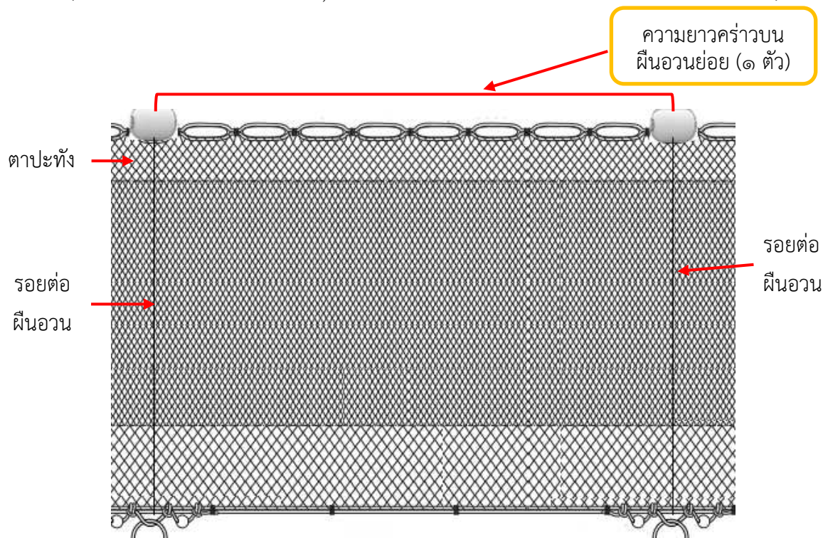
ภาพที่ ๒ ลักษณะผืนอวนย่อยของอวนล้อมจับและตำแหน่งการวัดความยาว
