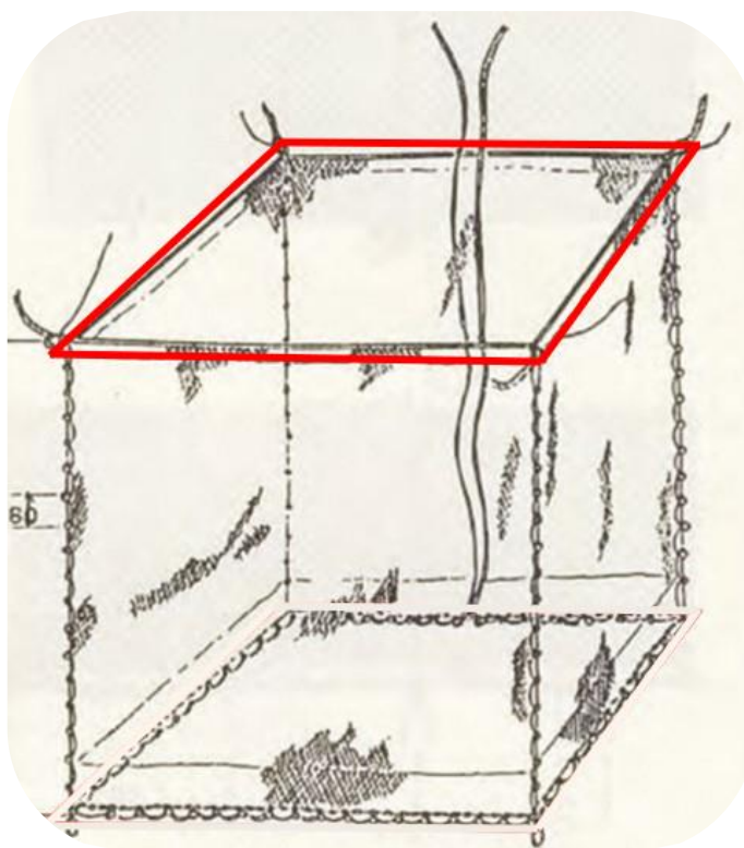
ภาพที่ ๕๖ ลักษณะของเครื่องมืออวนครอบปลาเกตุขณะปล่อยอวนเพื่อจับสัตว์น้ำ (กรมประมง, ๒๕๔๐)
