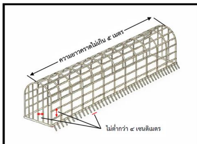
ภาพที่ ๓๙ วิธีการวัดคราดปลิงทะเลแบบตะแกรงซี่คราด
