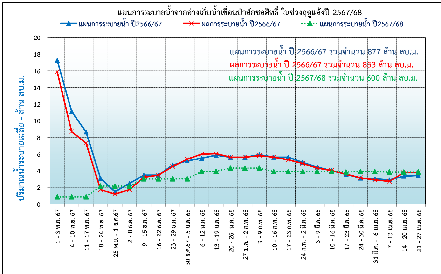
รูปที่ 3 กราฟแสดงแผนการระบายน้ำจากอ่างเก็บน้ำเขื่อนป่าสักชลสิทธิ์ ในช่วงฤดูแล้ง ปี 2567/68
