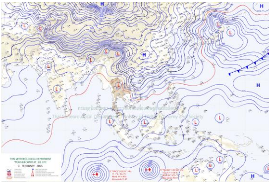
แผนที่อากาศผิวพื้น 4 กุมภาพันธ์ 2568 เวลา 01:00
